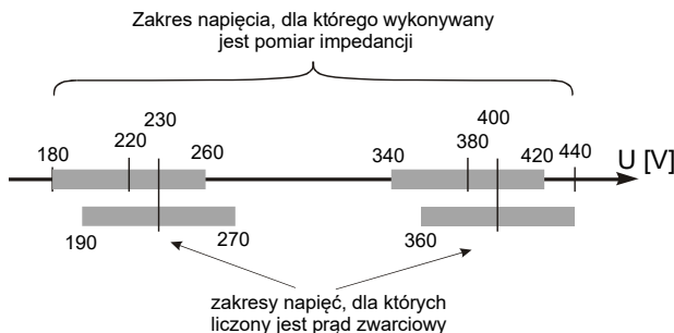
Rys.20. Zależności między napięciem sieci a możliwością wyliczenia prądu zwarciovowego
